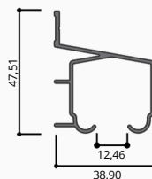
Trilho Convexo c/ Aba
