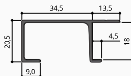
Perfil 18
