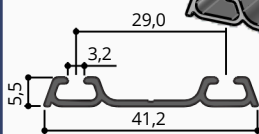
Trilho Inferior para Portas de Passagem
