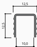
Trilho Inferior para Portas de Passagem
