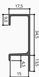
Trilho Inferior 29
